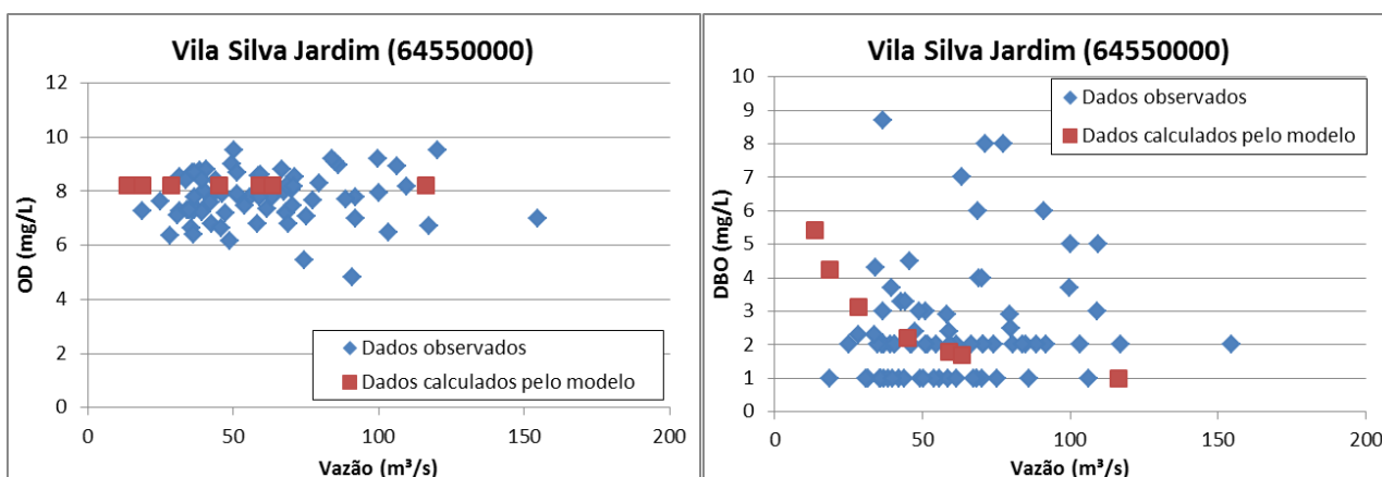
Figura 3. Comparação entre as concentrações de OD e DBO observadas na estação de monitoramento Vila Silva Jardim no rio Pirapó e as calculadas pelo modelo
