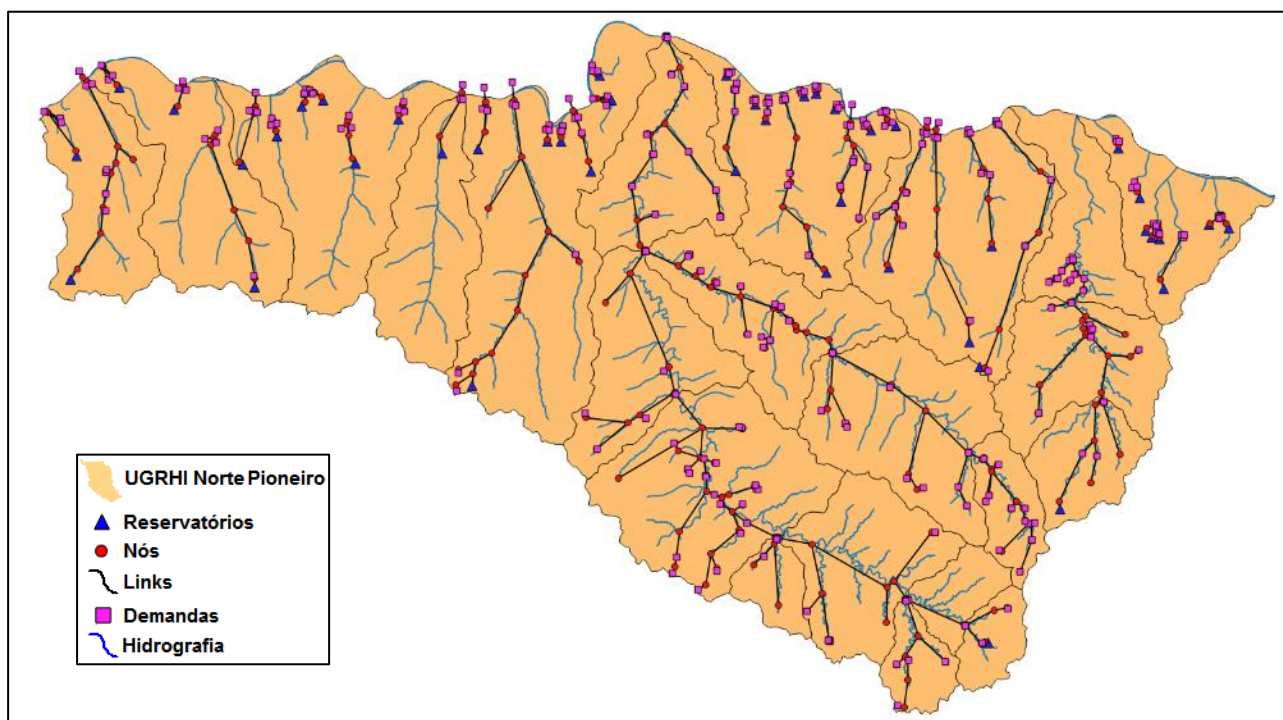
Figura 1. Rede de canais adotada no modelo Acquanet para simulações da qualidade da água da UGRHI Piraponema
