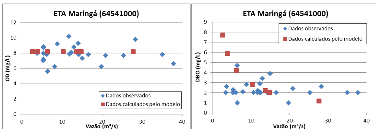
Figura 2. Comparação entre as concentrações de OD e DBO observadas na estação de monitoramento ETA Maringá no rio Pirapó e as calculadas pelo modelo
