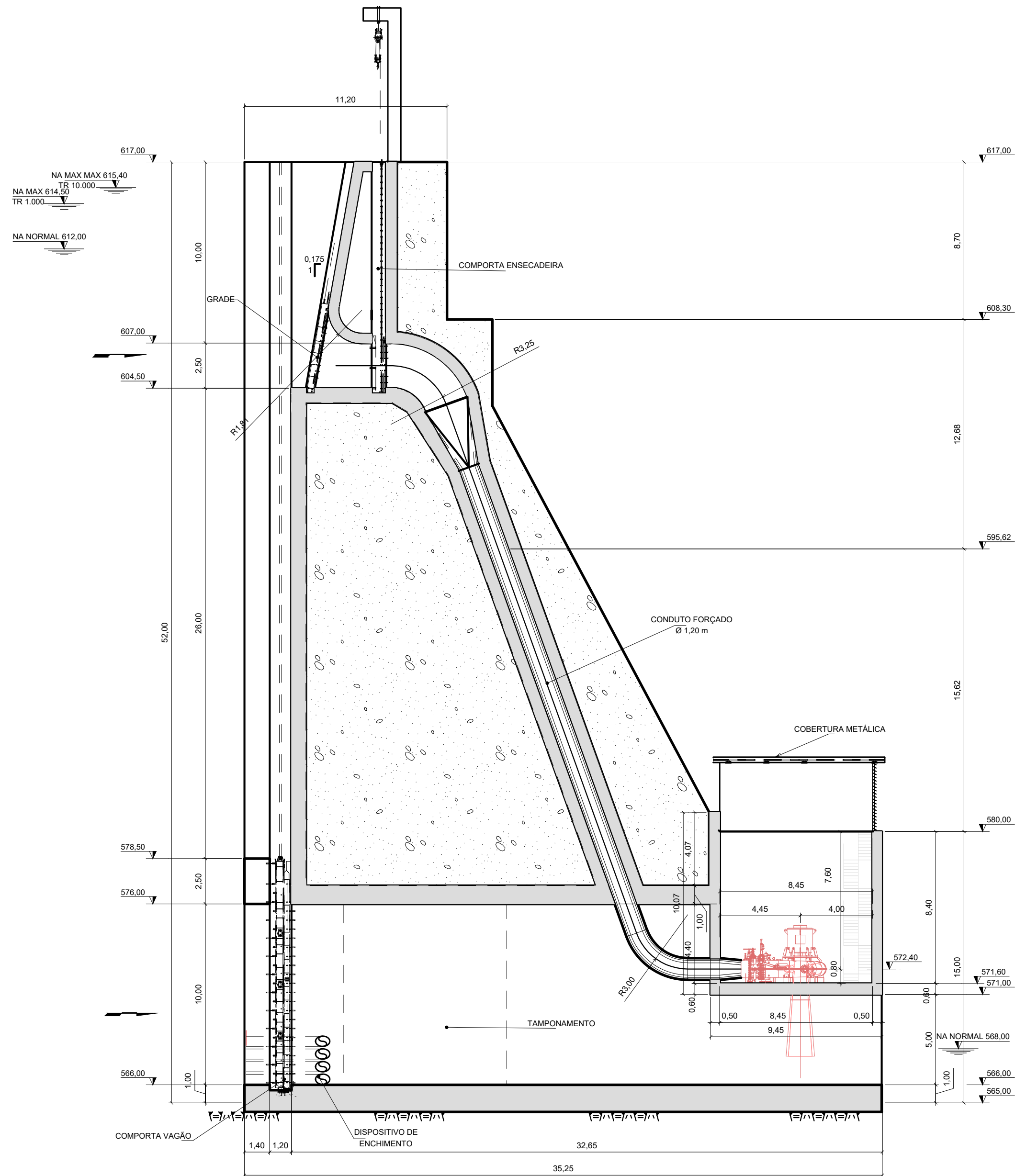
SEÇÃO - C Esc: 1:200
