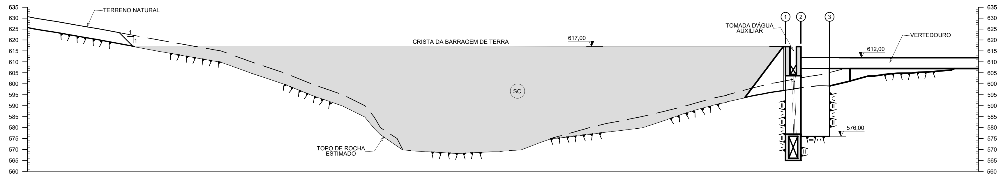
SEÇÃO - A Esc. 1:750 BPDE-C05-0010
