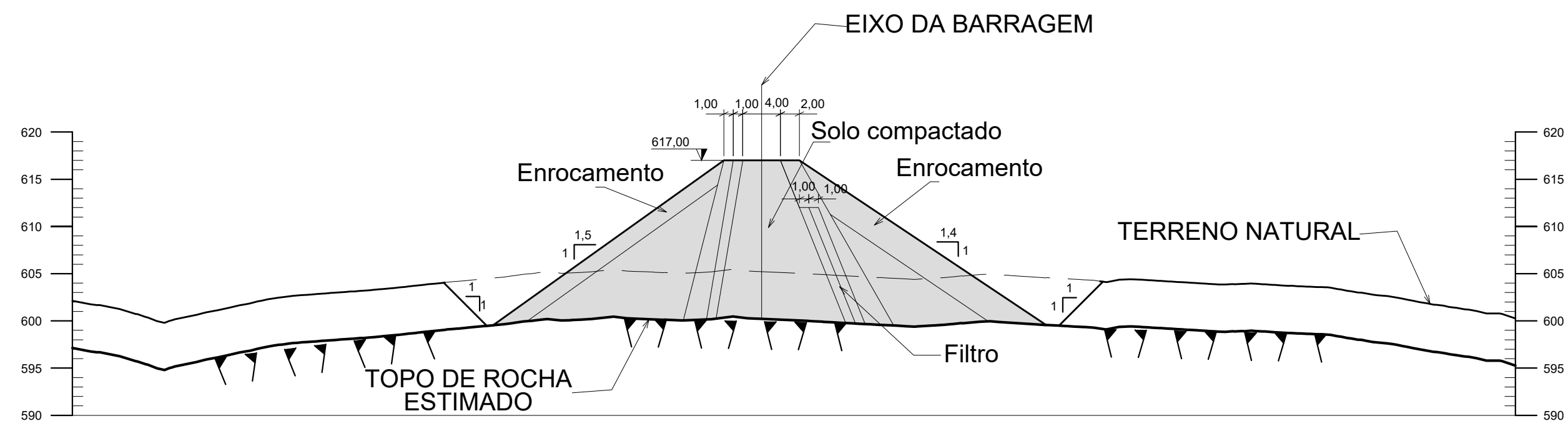
SEÇÃO - B Esc. 1:325 PBDE-C05-0010
