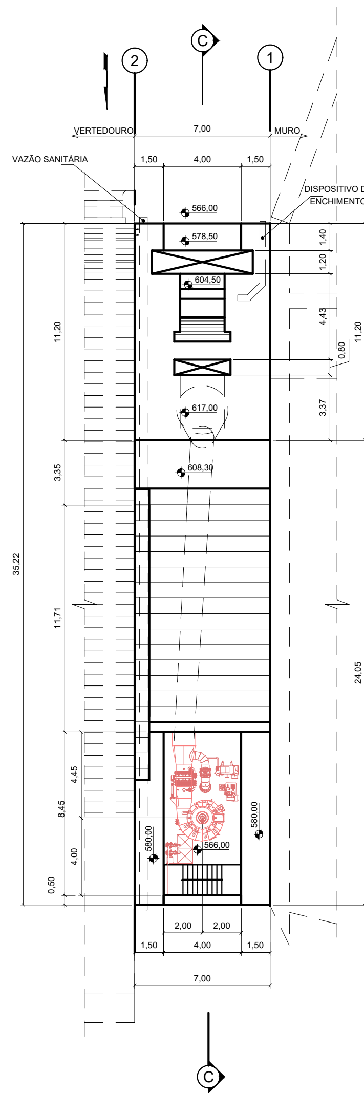
PLANTA EL.617,00 Esc: 1:200
