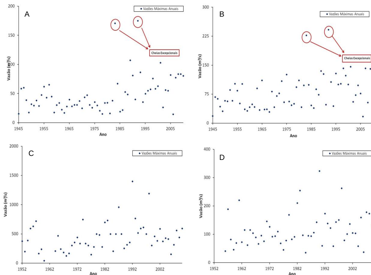
Figura 31: A- Vazões máximas no posto Porto Vitória (653650000), B- Vazões máximas no posto Fazenda Maracanã (65415000), C- Vazões máximas no posto Usina Cavernoso (65855000) e D- Vazões máximas no posto Ponte do Vitorino (65945000)
