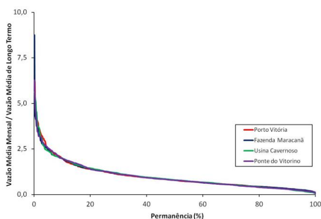
Figura 27: Curva de permanência dos postos analisados
