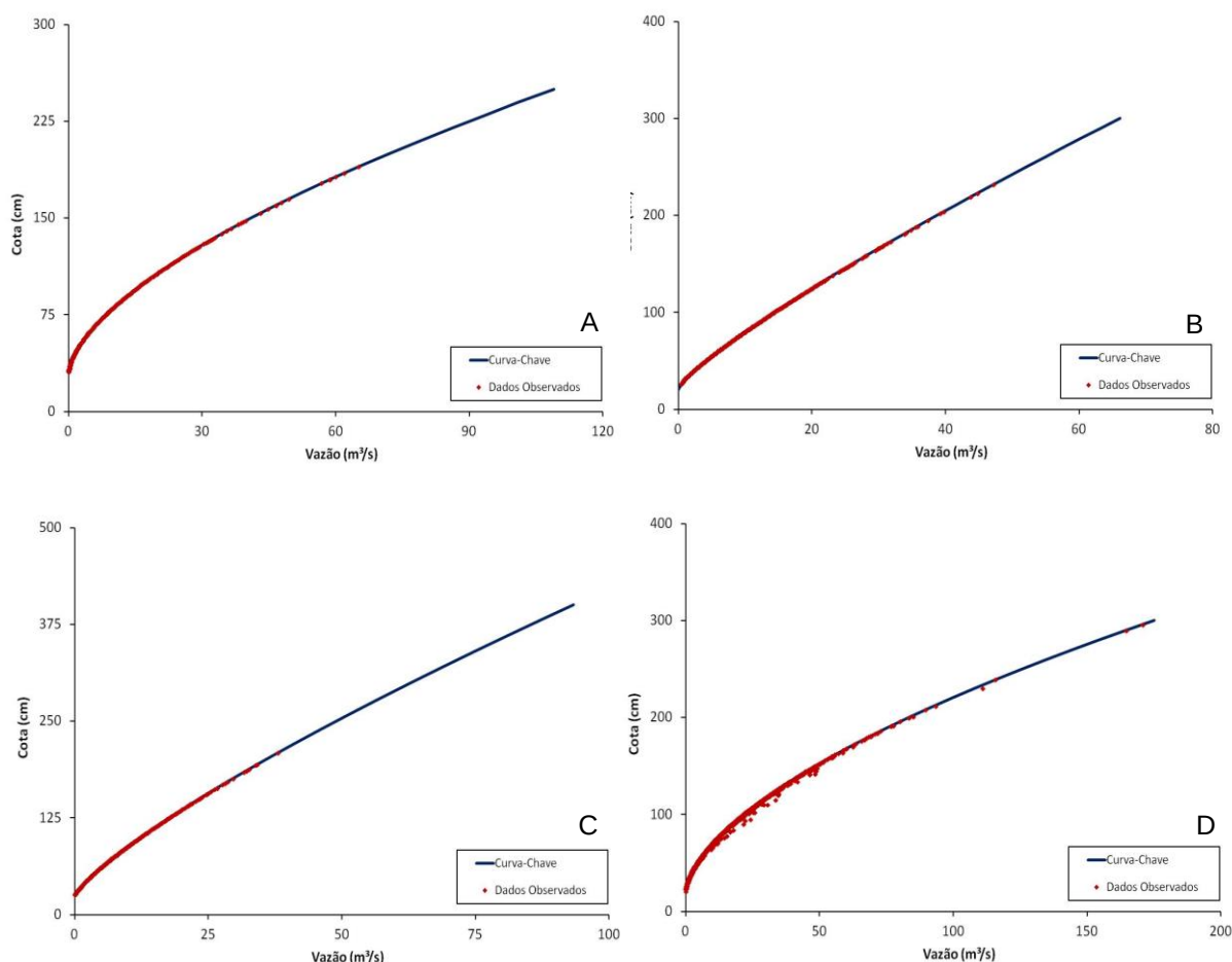
Figura 22: Curva-chave do Posto Porto Vitória, A- Período de Nov/45 a Abr/59, B-Período de Abr/45 a Dez/75, C- Período de Jan/76 a Dez/82 e D- Jan/83 a Dez/10
