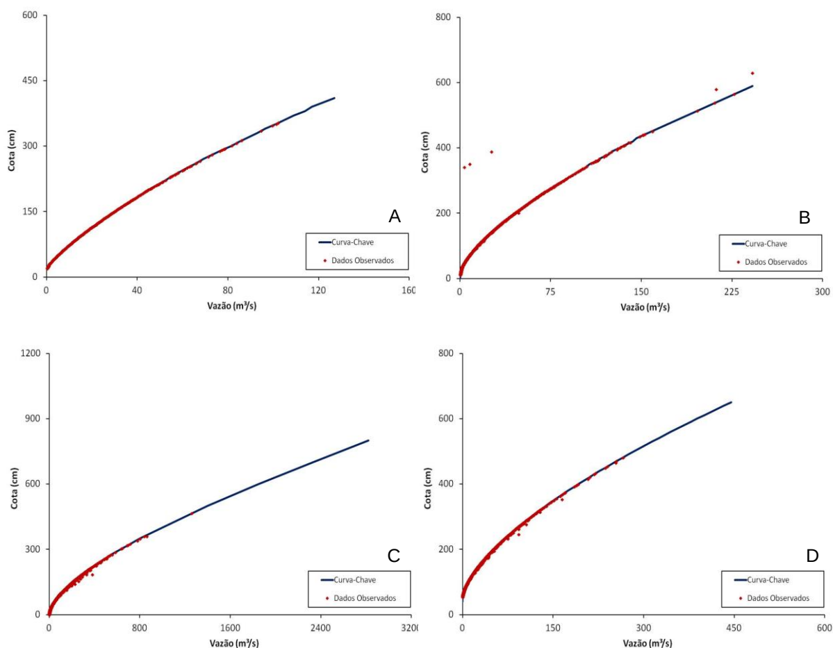
Figura 23: A- Curva-chave do Posto Fazenda Maracanã no período de Nov/45 a Ago/60, B- Curva-chave do Posto Fazenda Maracanã no período de Ago/60 a Dez/10, C- Curva-chave do Usina Cavernoso no período de Jan/52 a Dez/10 e D- Curva-chave posto Ponte do Vitorino no período de Jul/56 a Dez/10
