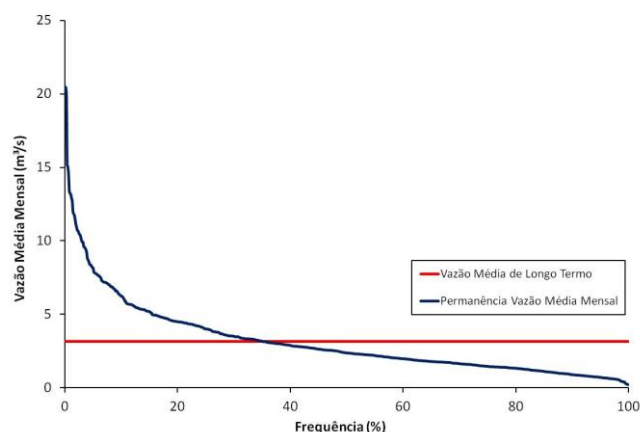
Figura 30: Curva de permanência vazões médias mensais – CGH Cão Menor.
