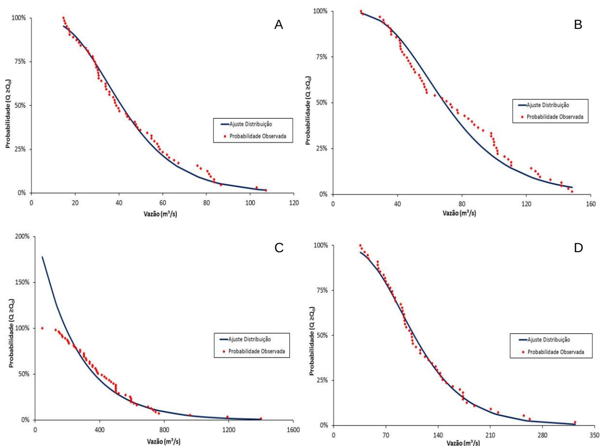
Figura 32: A - Ajuste distribuição Gumbel - posto Porto Vitória (65365000), B- Ajuste distribuição Gumbel - posto Fazenda Maracanã (65415000), C- Ajuste distribuição Gumbel - posto Usina Cavernoso (65855000) e D- Ajuste distribuição Gumbel - posto Ponte do Vitorino (65945000)
