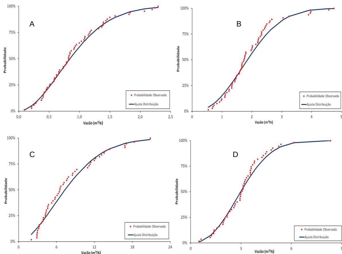
Figura 35: Ajuste distribuição Weibull, A- posto Porto Vitória (65365000), B- posto Fazenda Maracanã (65415000), C- posto Usina Cavernoso (65855000) e D Ajuste distribuição Gumbel para o posto Ponte do Vitorino (65945000)
