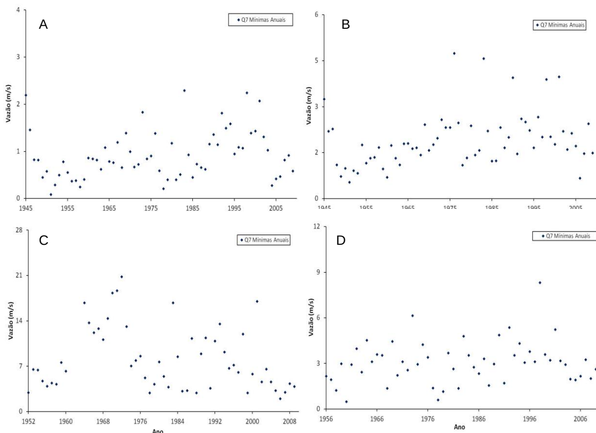
Figura 34: A - Vazões mínimas no posto Porto Vitória (653650000), B- Vazões mínimas no posto Fazenda Maracanã (65415000), C- Vazões mínimas no posto Usina Cavernoso (65855000) e D- Vazões mínimas no posto Ponte do Vitorino (65945000)
