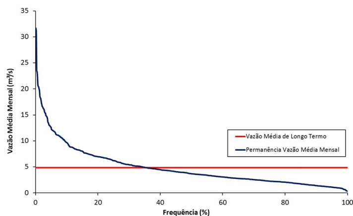
Figura 30: Curva de permanência vazões médias mensais – CGH Órion 2.
