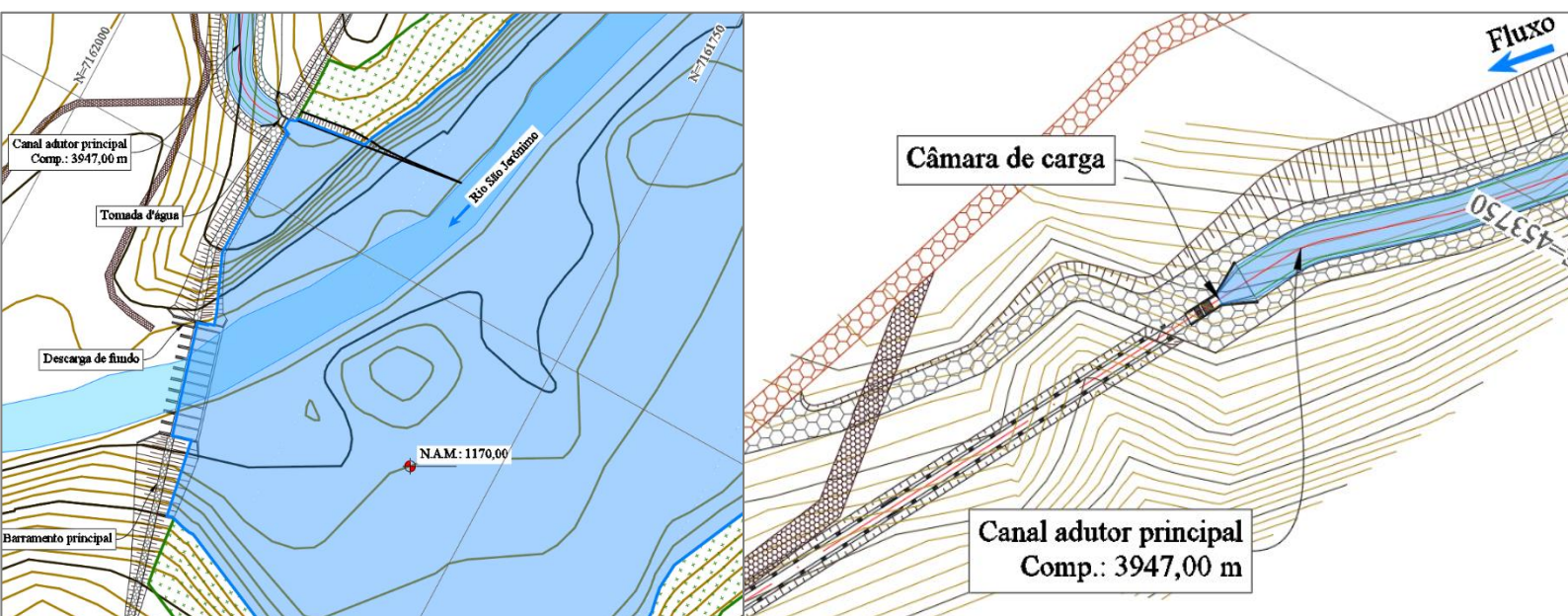
BARRAMENTO, CANAL ADUTOR PRINCIPAL E CÂMARA DE CARGA
