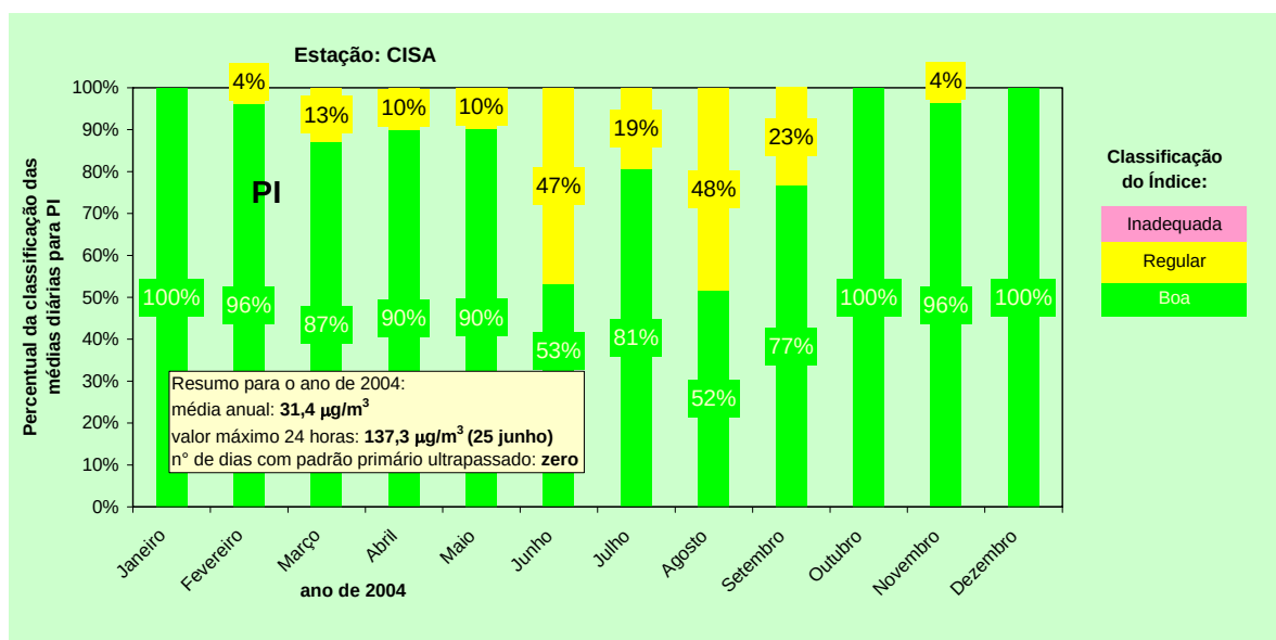
Gráfico 8: Classificação das médias diárias para PI na Estação CISA no ano de 2004
