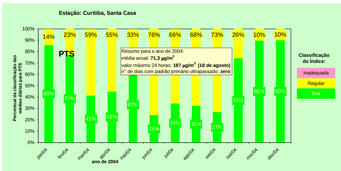
Gráfico 3: Classificação das médias diárias para PTS na Estação Santa Casa no ano de 2004
