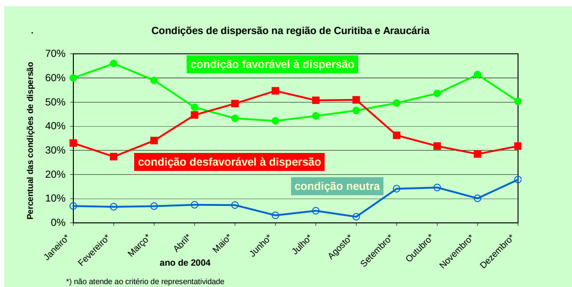
Gráfico 2: Condições de dispersão nas estações automáticas de monitoramento da qualidade do ar
