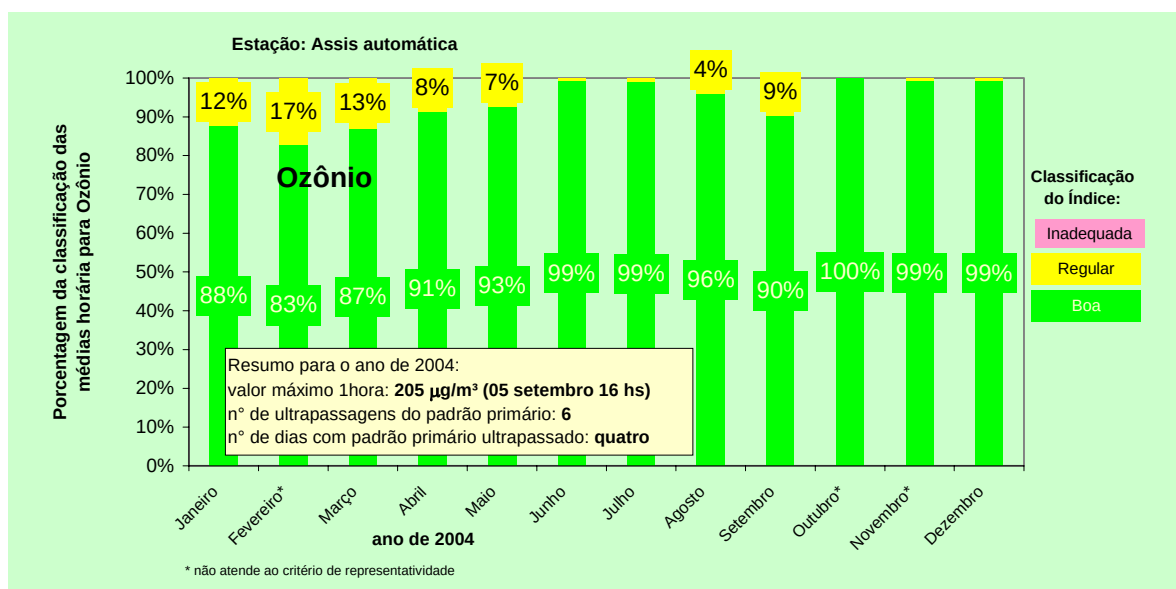
Gráfico 12: Classificação das médias horárias para Ozônio na Estação Assis automática
