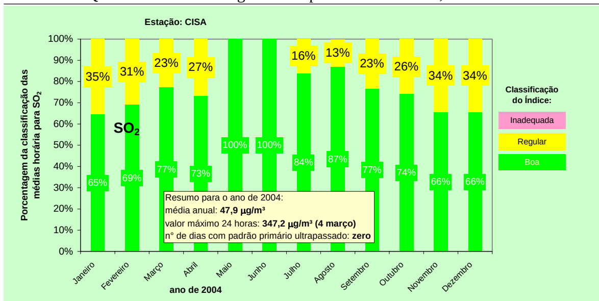
Gráfico 10: Classificação das médias diárias para SO 2 na Estação CISA no ano de 2004
