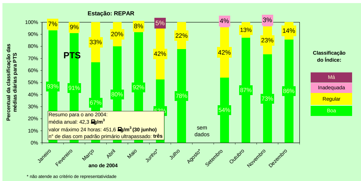
Gráfico 6: Classificação das médias diárias para PTS na Estação REPAR no ano de 2004
