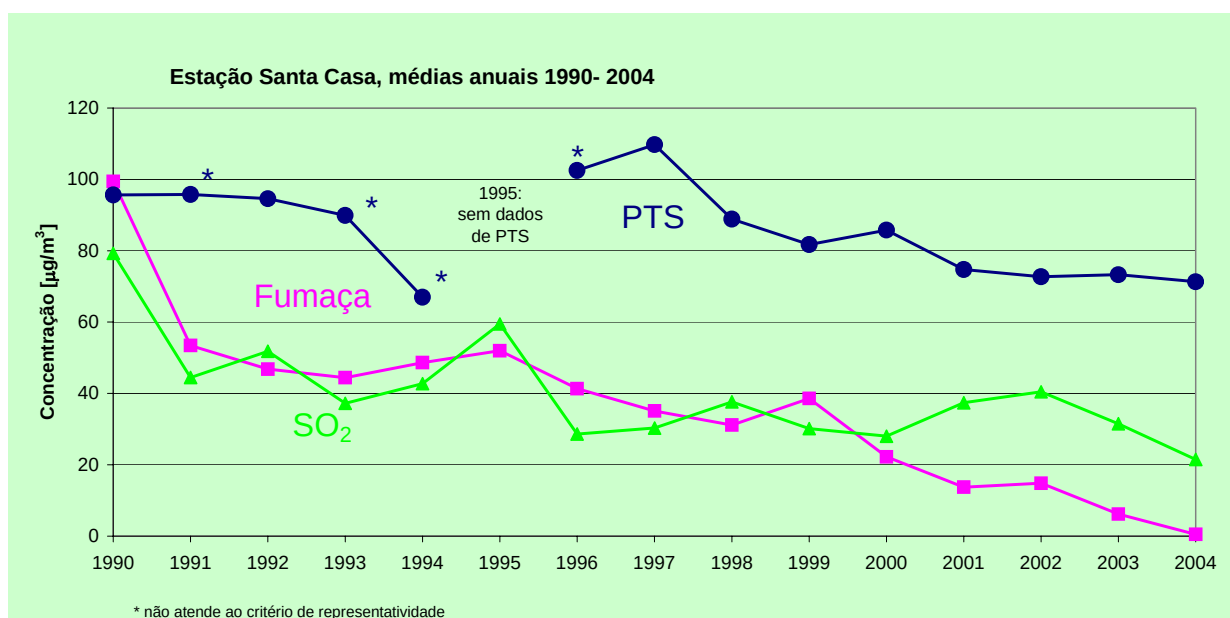
Gráfico 9: Médias anuais para SO 2 , Fumaça e PTS no período de 1990 até 2004 na Estação Santa Casa
