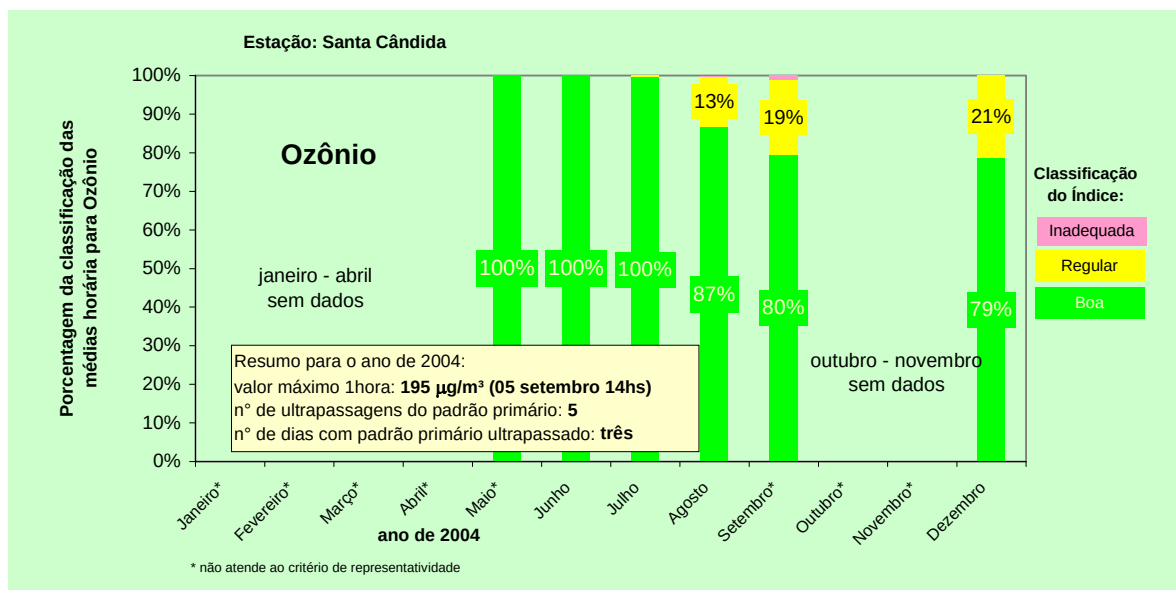
Gráfico 11: Classificação das médias horárias para Ozônio na Estação Santa Cândida
