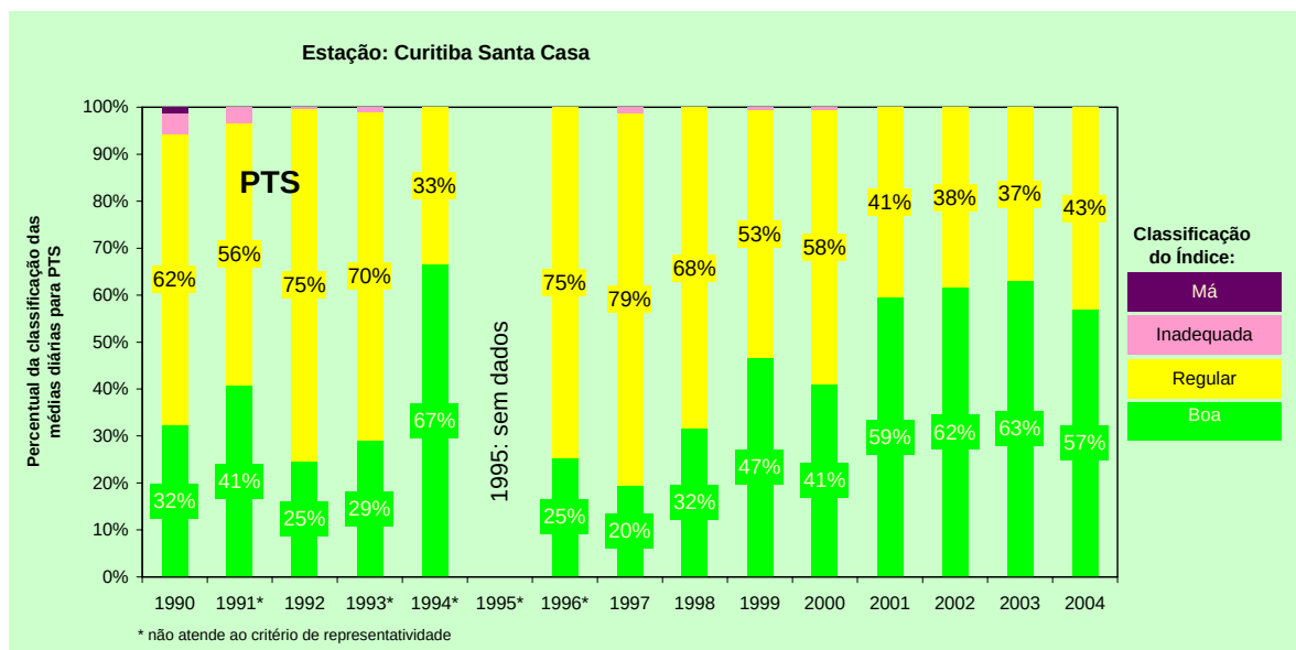
Gráfico 4: Classificação das médias diárias para PTS na Estação Santa Casa entre 1990-2004
