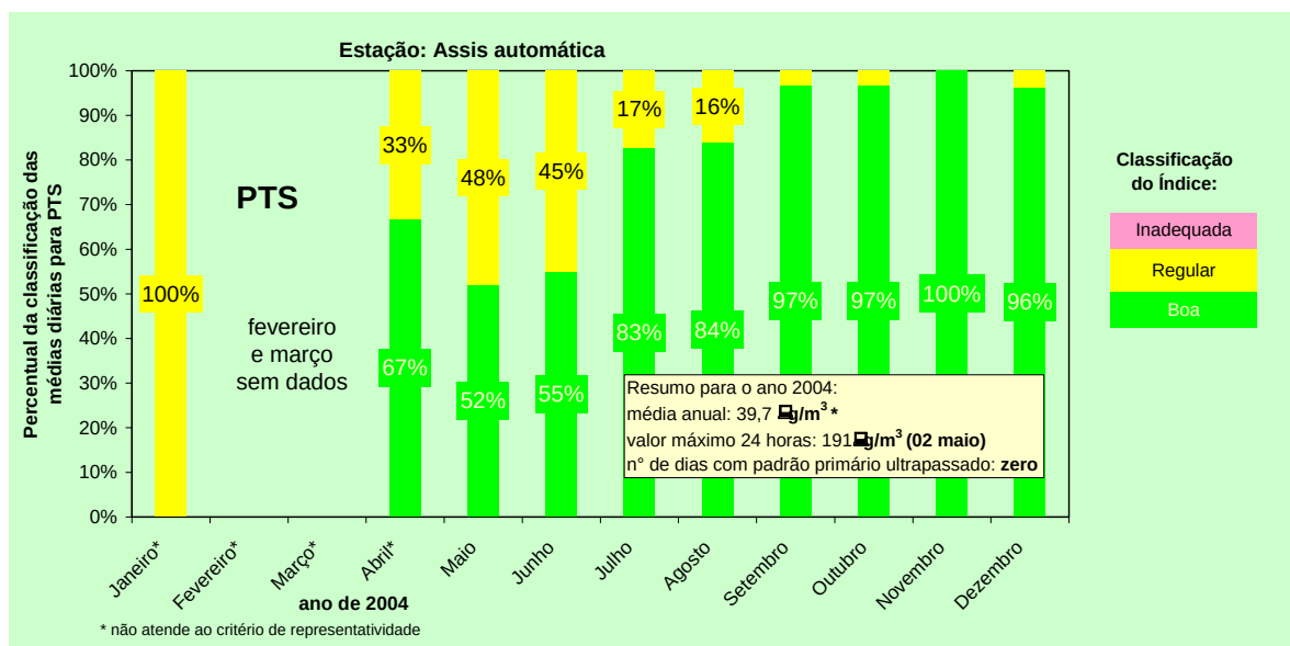
Gráfico 5: Classificação das médias diárias para PTS na Estação Araucária Assis automática no ano de 2004
