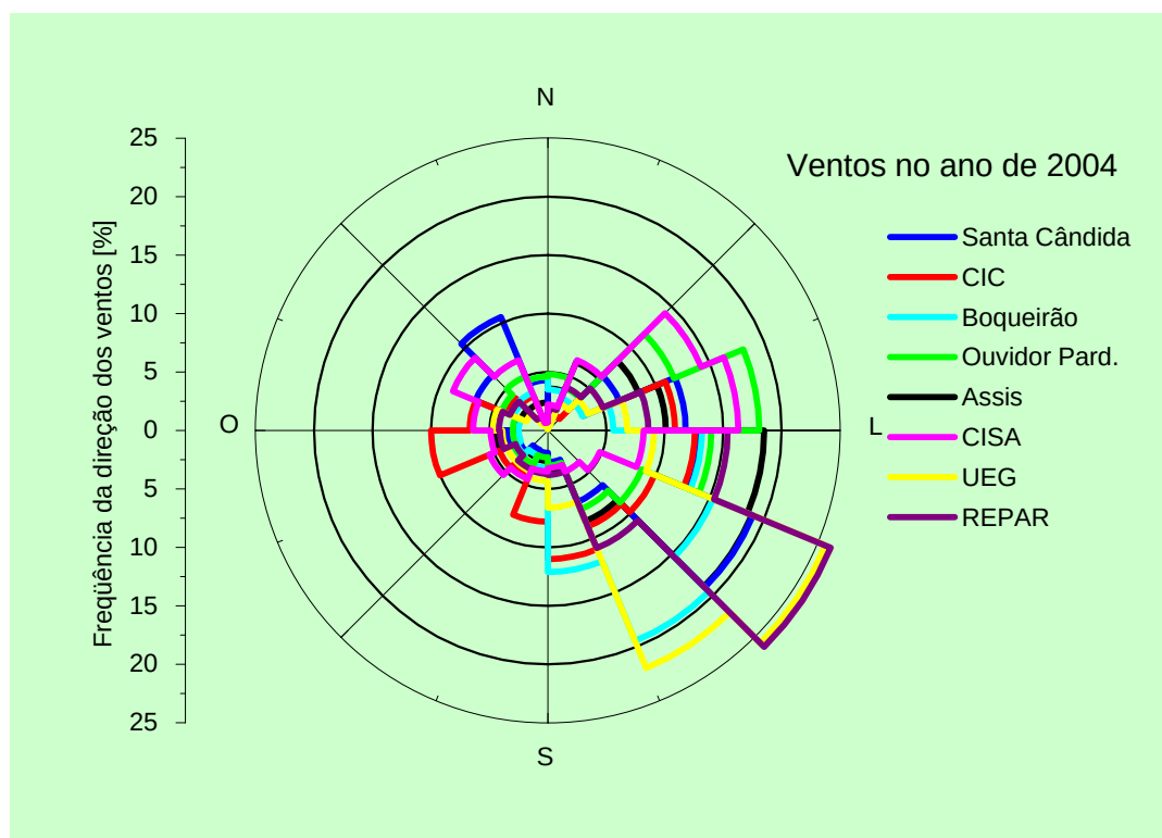
Gráfico 1: Frequência dos ventos nas estações automáticas de monitoramento da qualidade do ar
