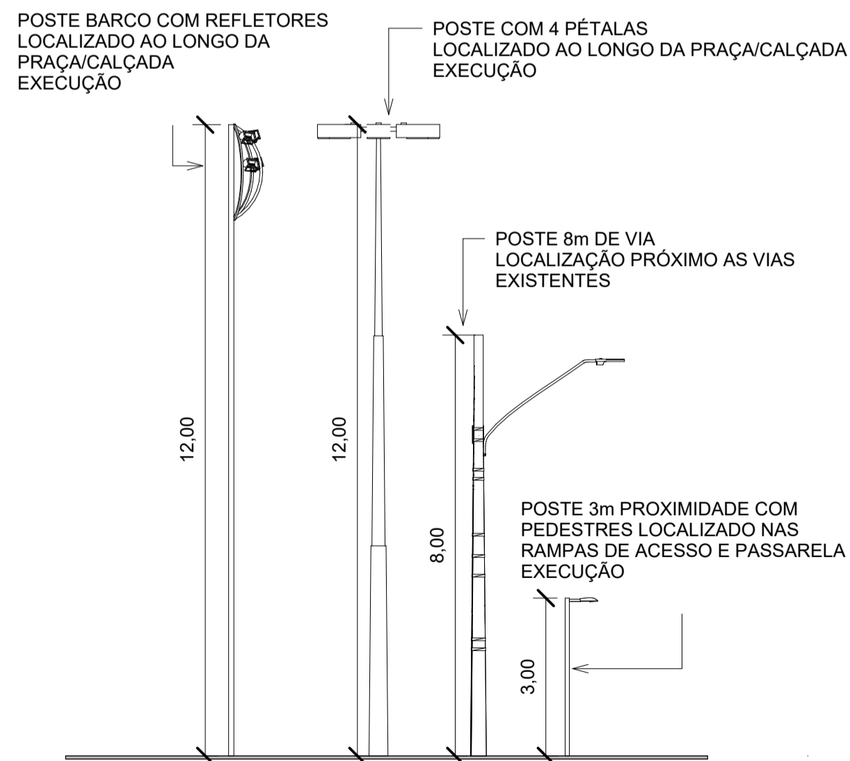
3 DETALHE POSTES 1 : 100
