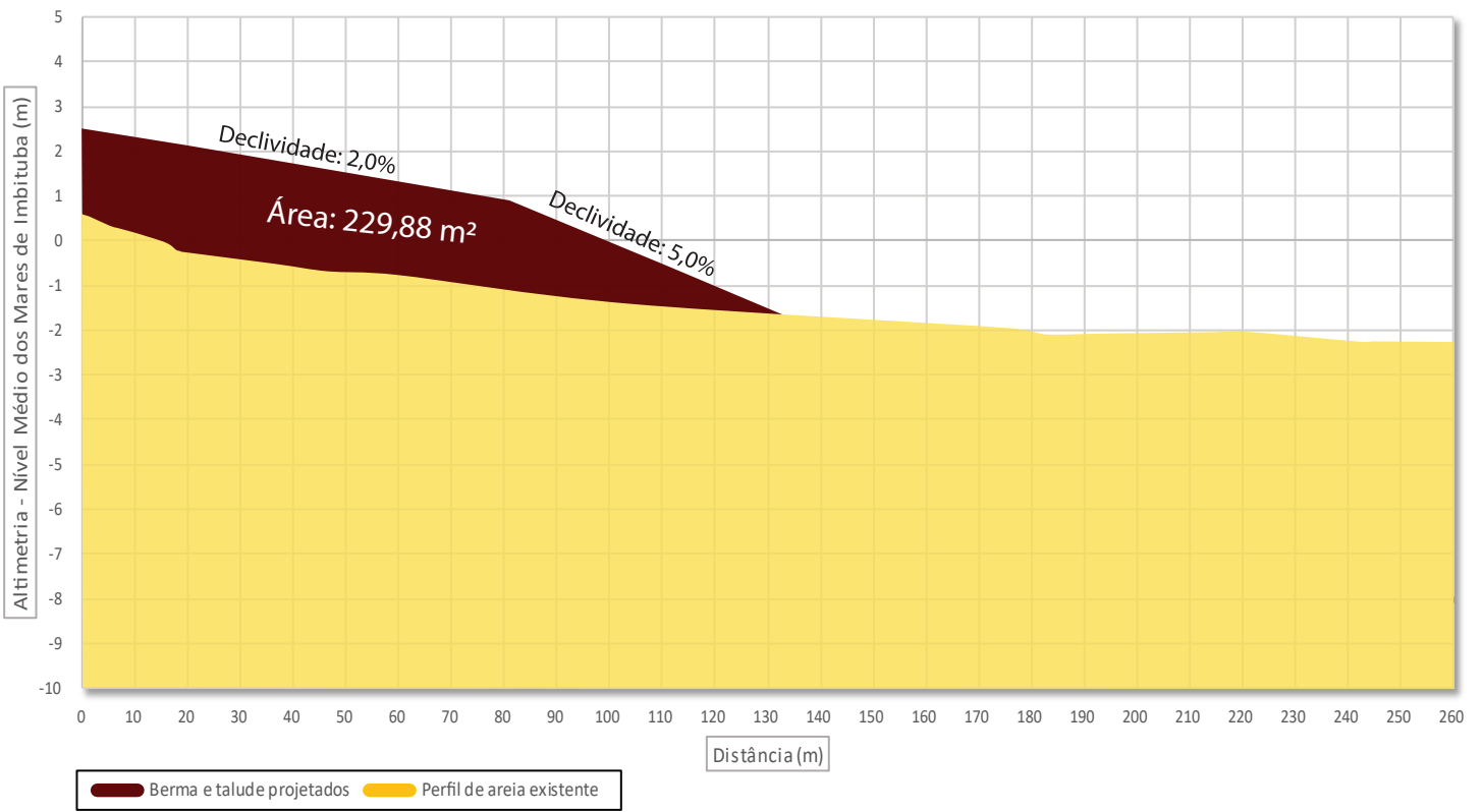
Caieras - Seção 1
