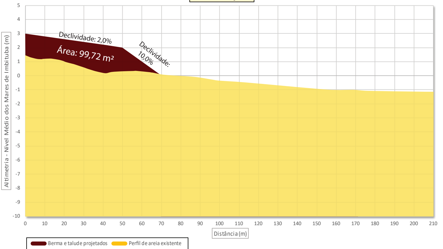
Caieiras- Seção 5
