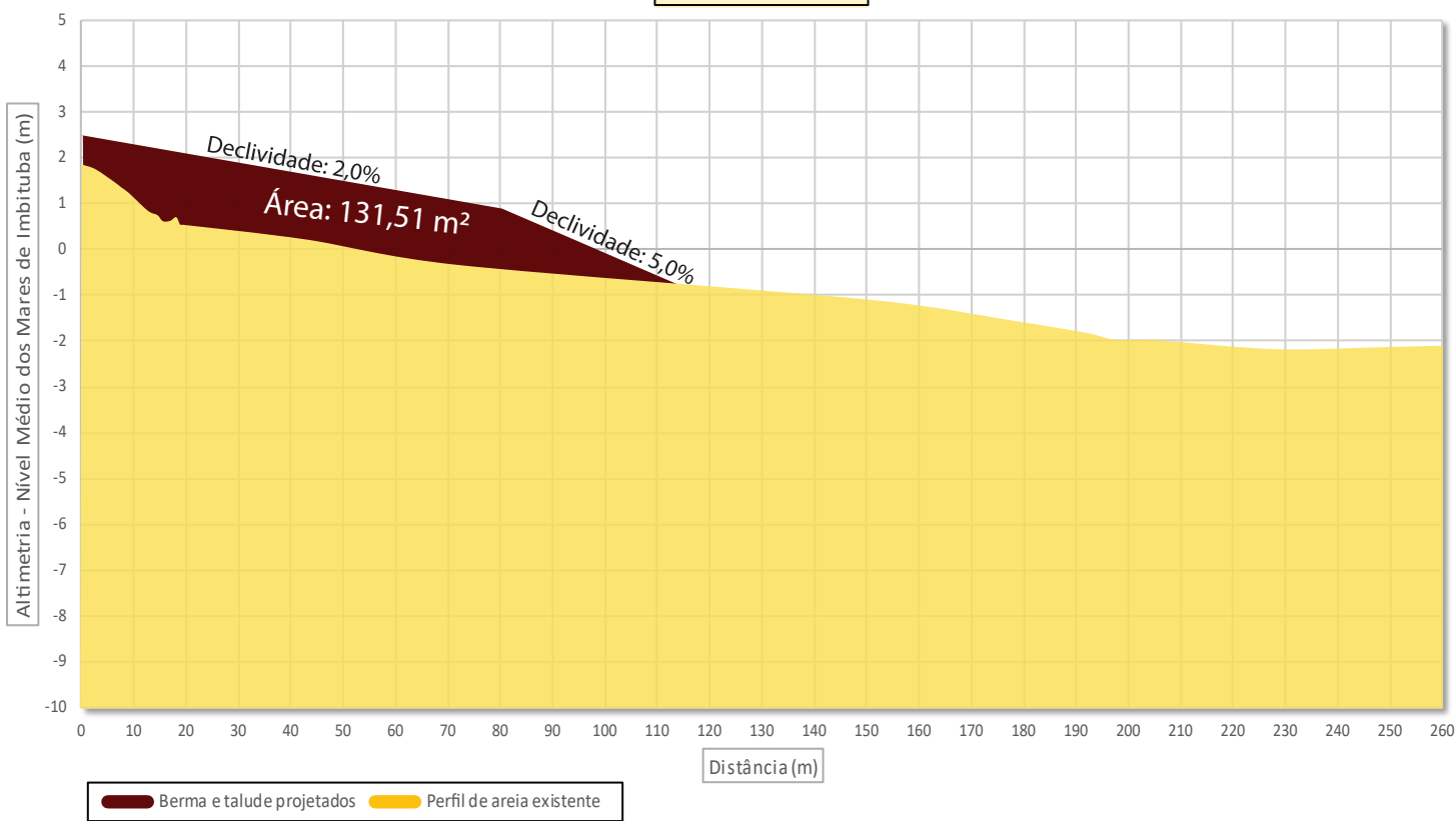
Caieiras - Seção 2
