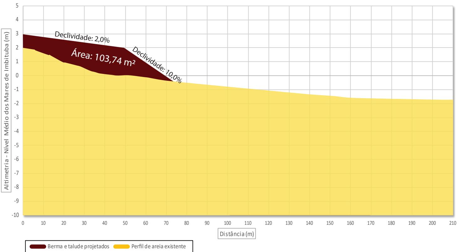
Caieiras- Seção 6
