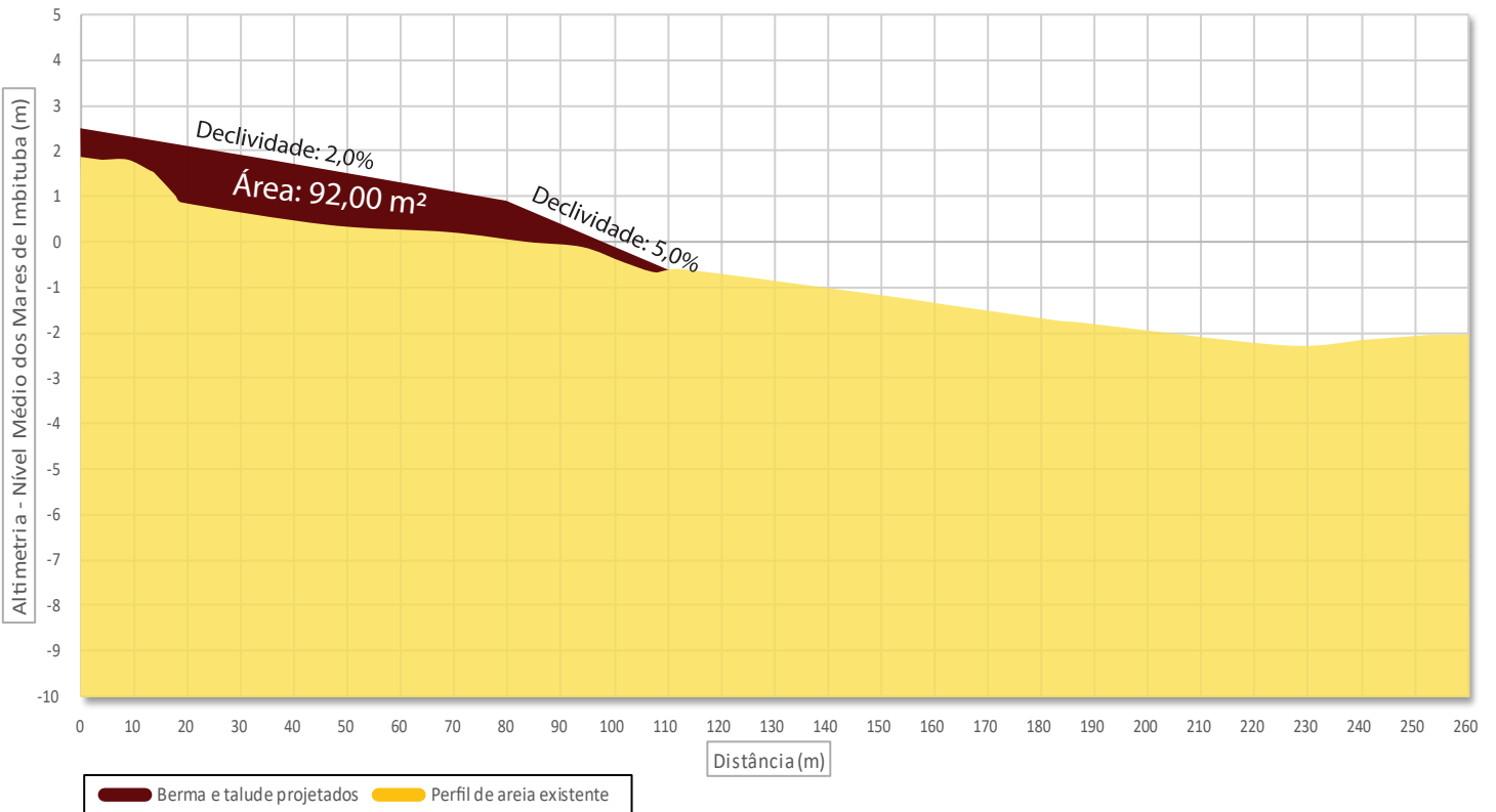
Caieiras - Seção 3
