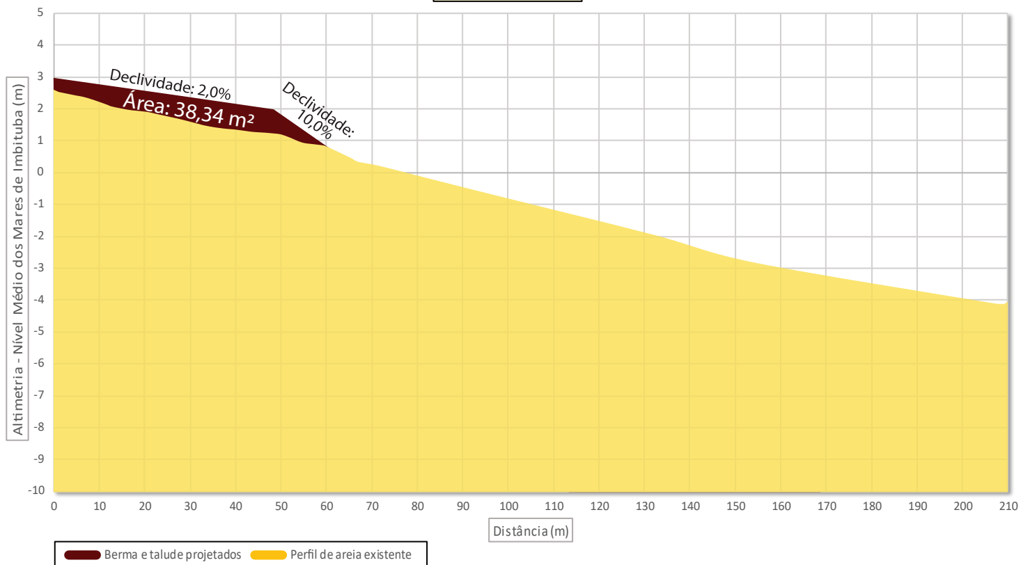
Caieras - Seção 7
