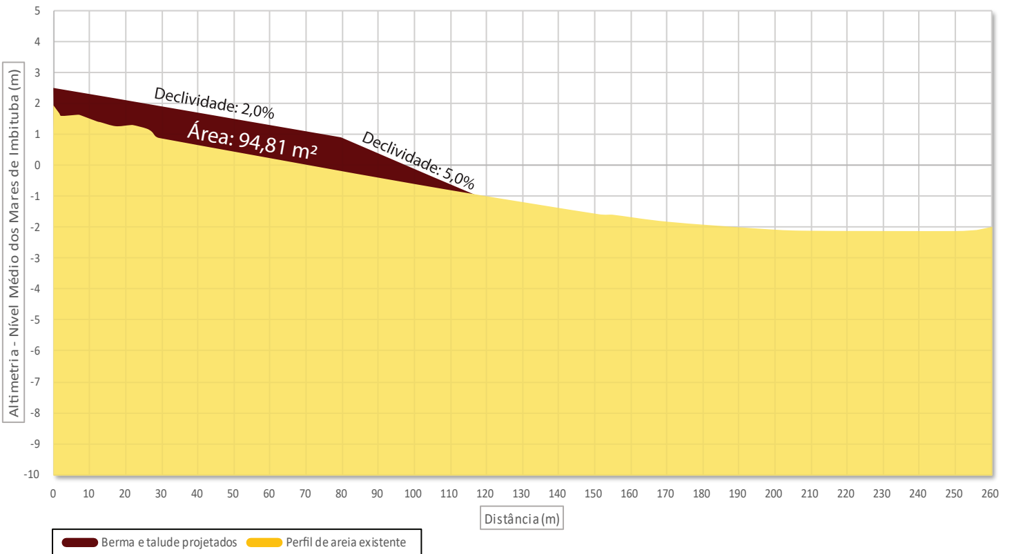
Caieiras - Seção 4
