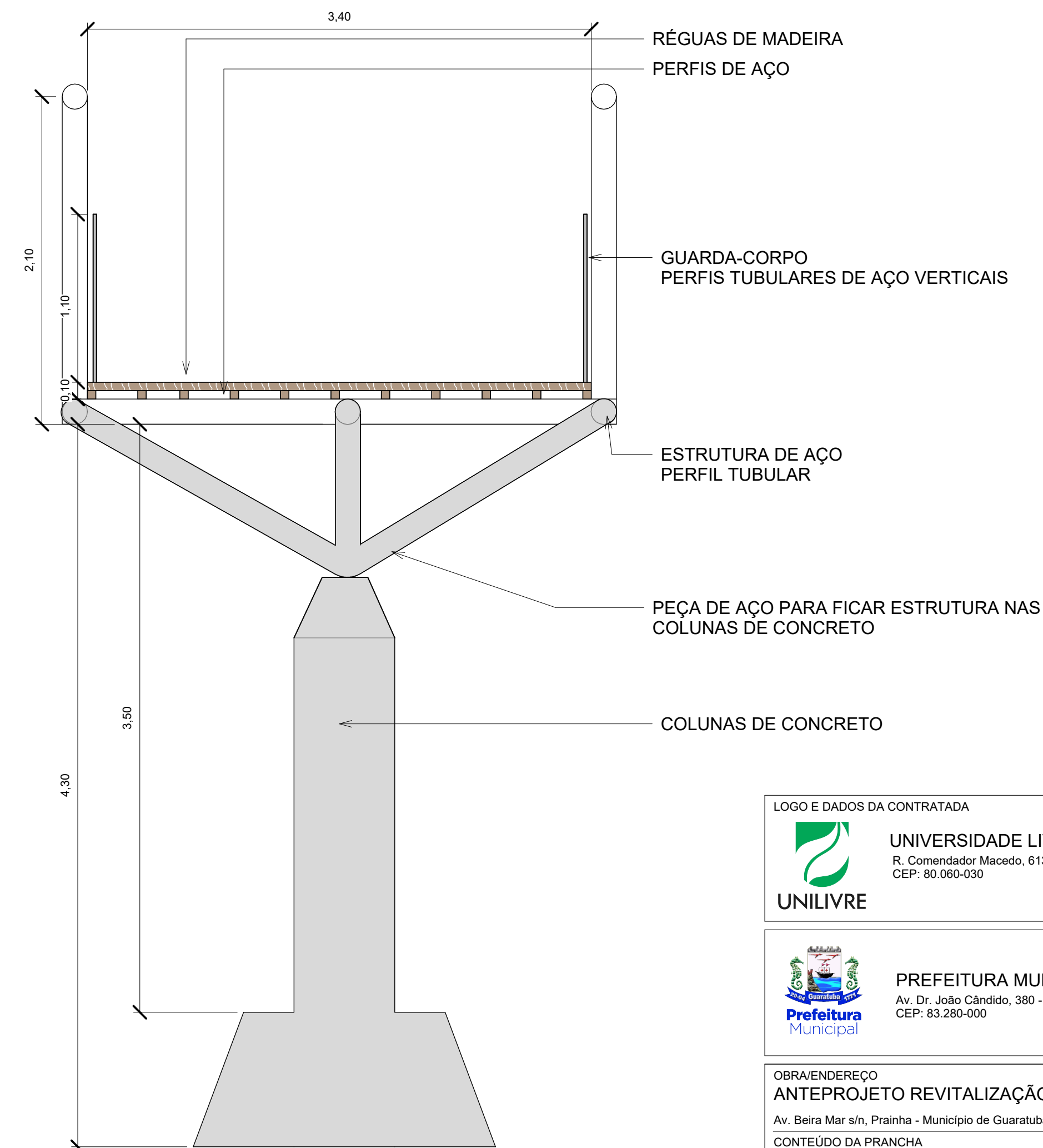
3 DETALHE PILARES PASSARELAS PEDONAIS 1 : 25
