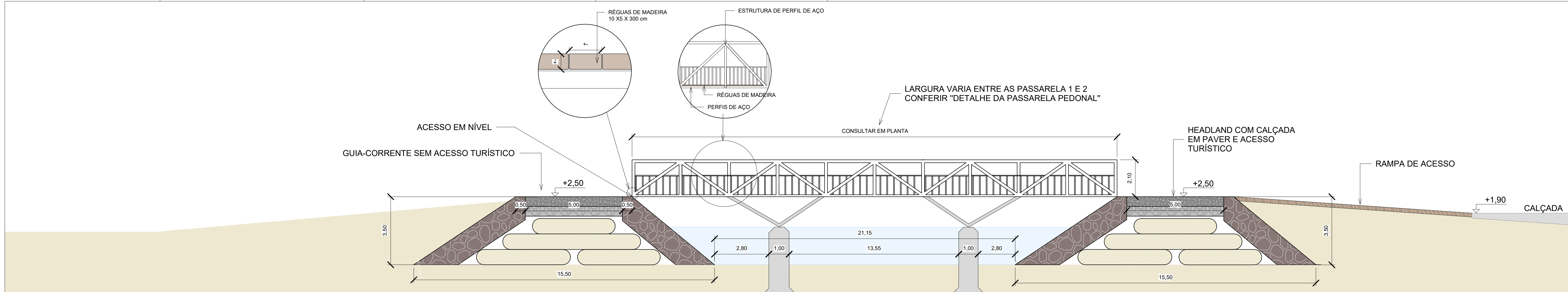
1 CORTE LONGITUDINAL PASSARELA PEDONAL 1 : 100
