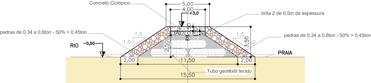
Estaca 06
