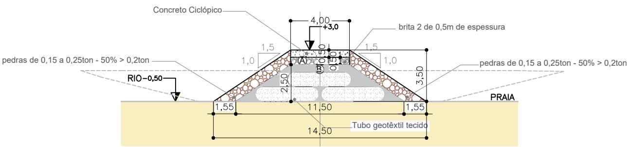
Estaca 02
