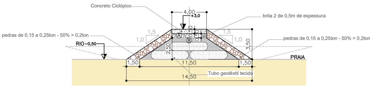
Estaca 00
