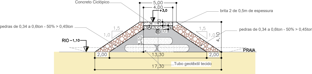
Estaca 07+10 – CABEÇO
