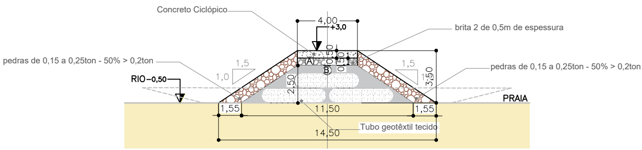
Estaca 04
