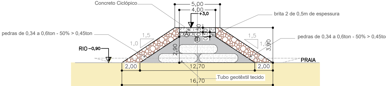
Estaca 07
