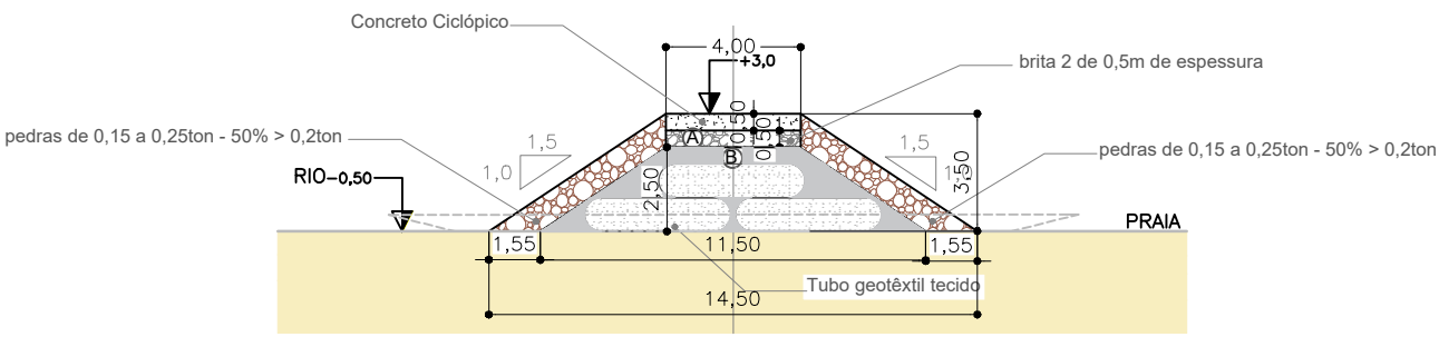
Estaca 05M
