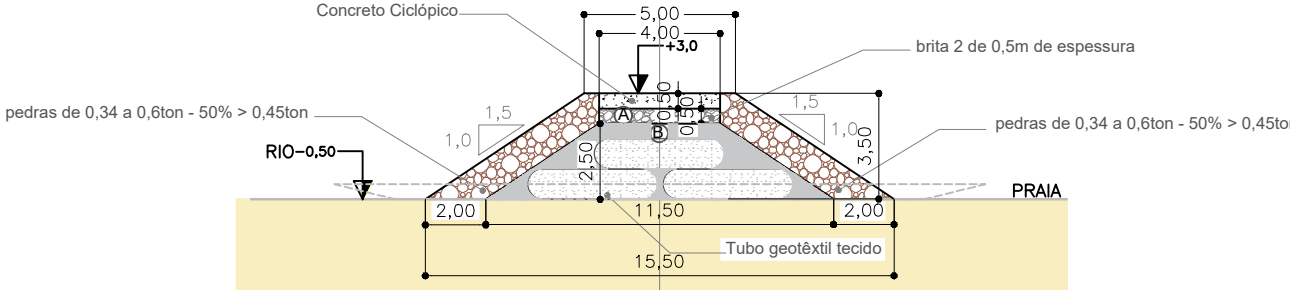
Estaca 05J
