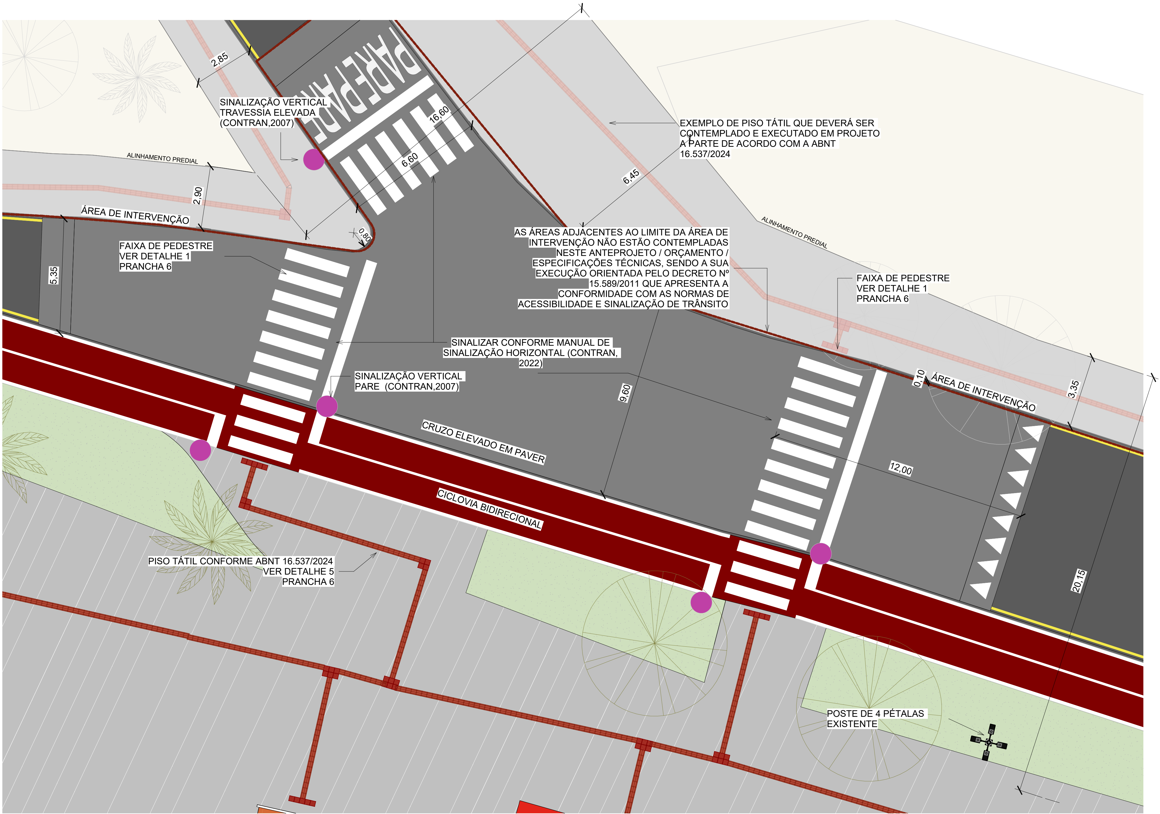
6 DETALHE ENCONTRO VIÁRIO 6 1 : 100
