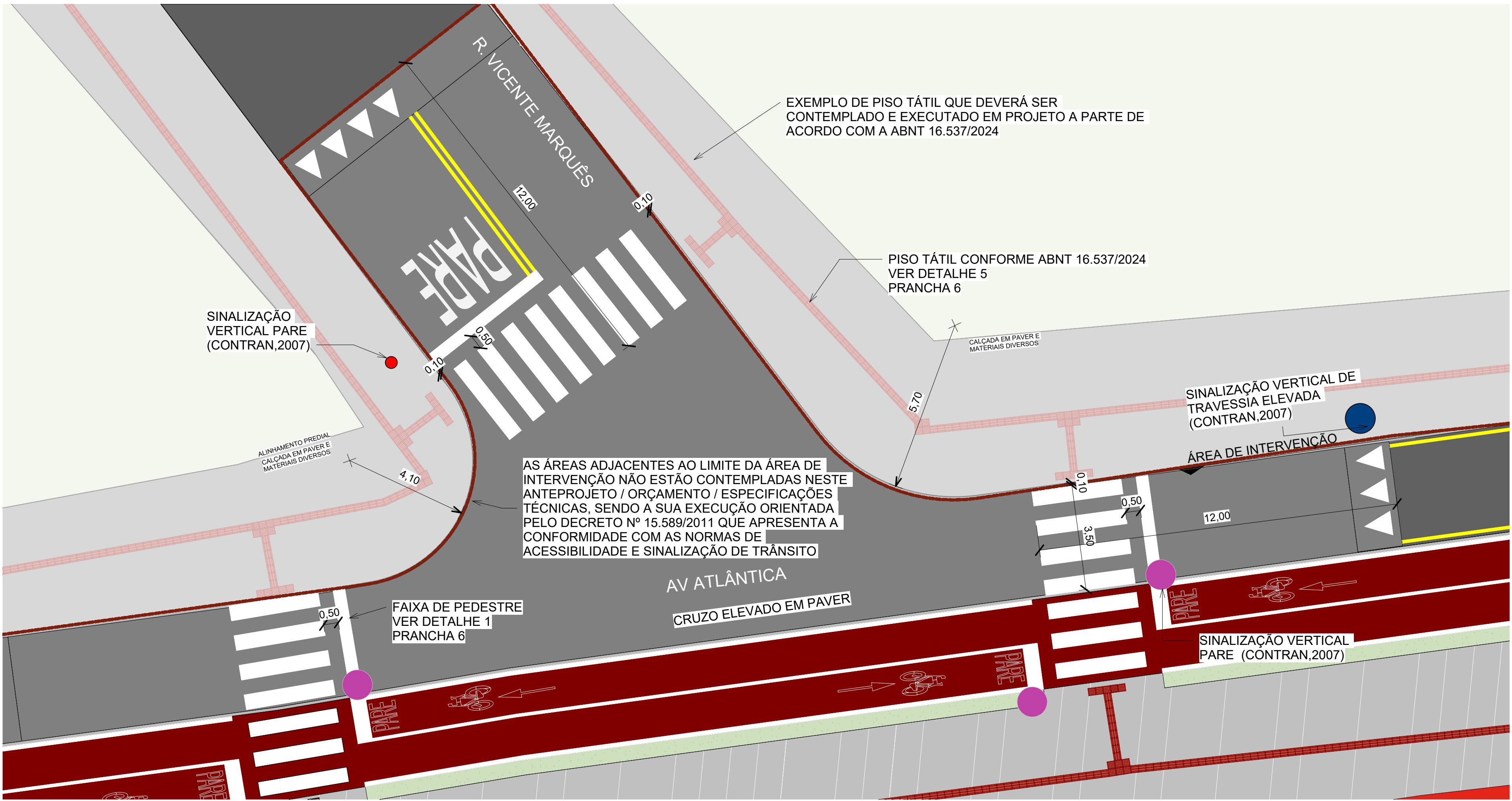
4 ENCONTRO VIÁRIO 4 1 : 100
