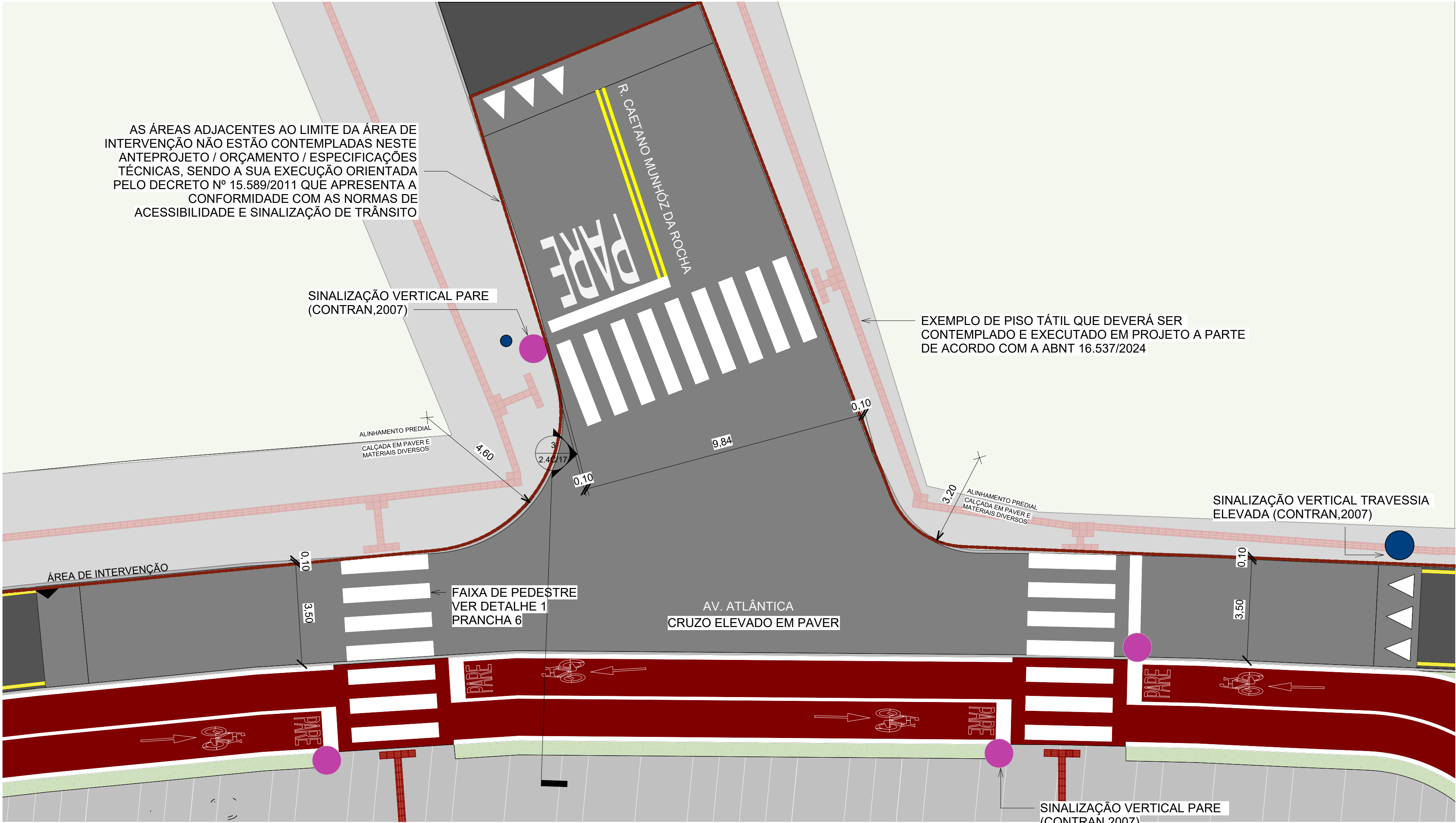
3 ENCONTRO VIÁRIO 3 1 : 100
