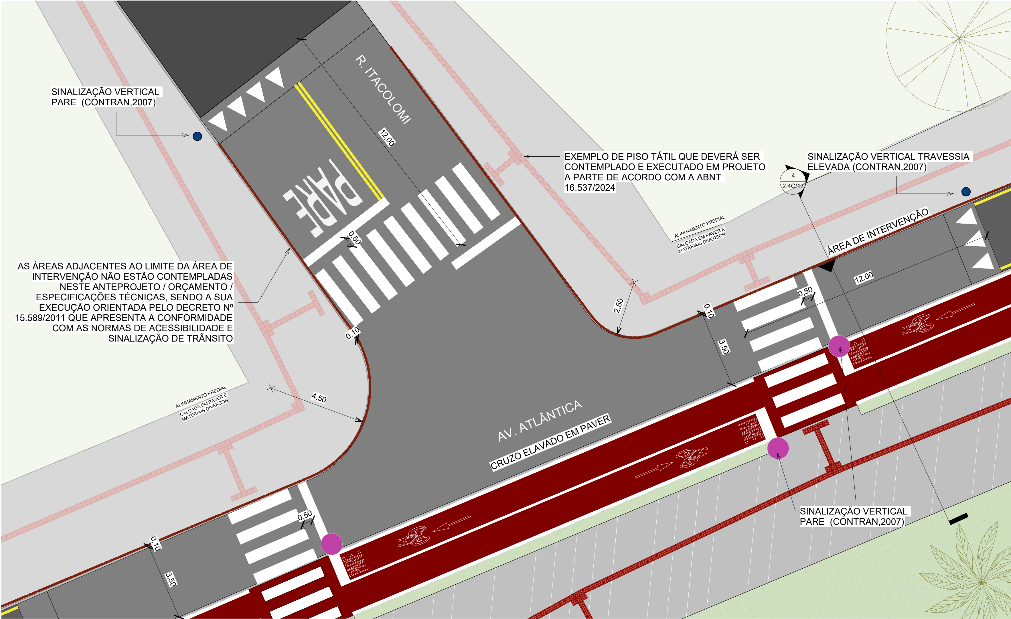
5 ENCONTRO VIÁRIO 5 1 : 100
