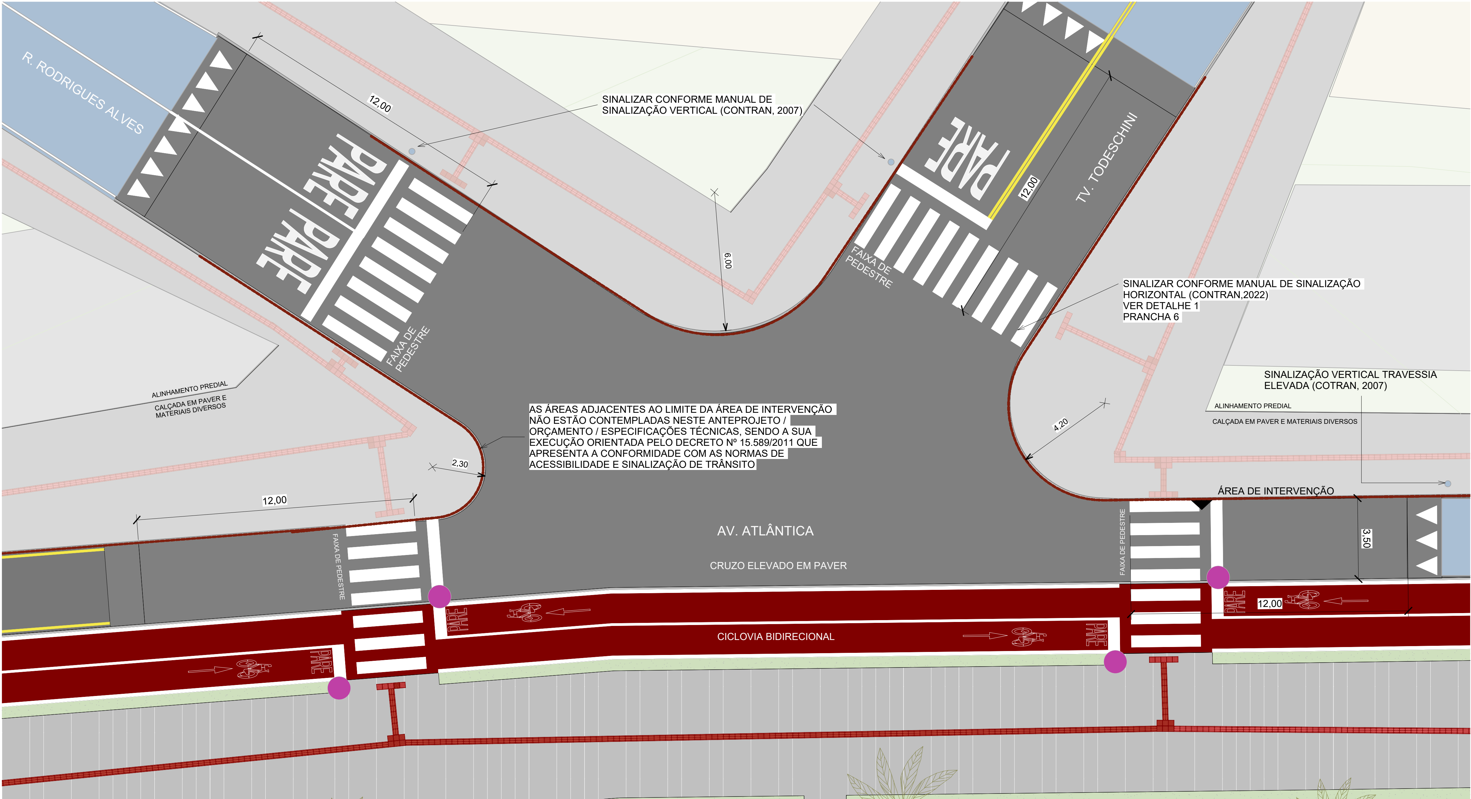
1 ENCONTRO VIÁRIO 1 1 : 100
