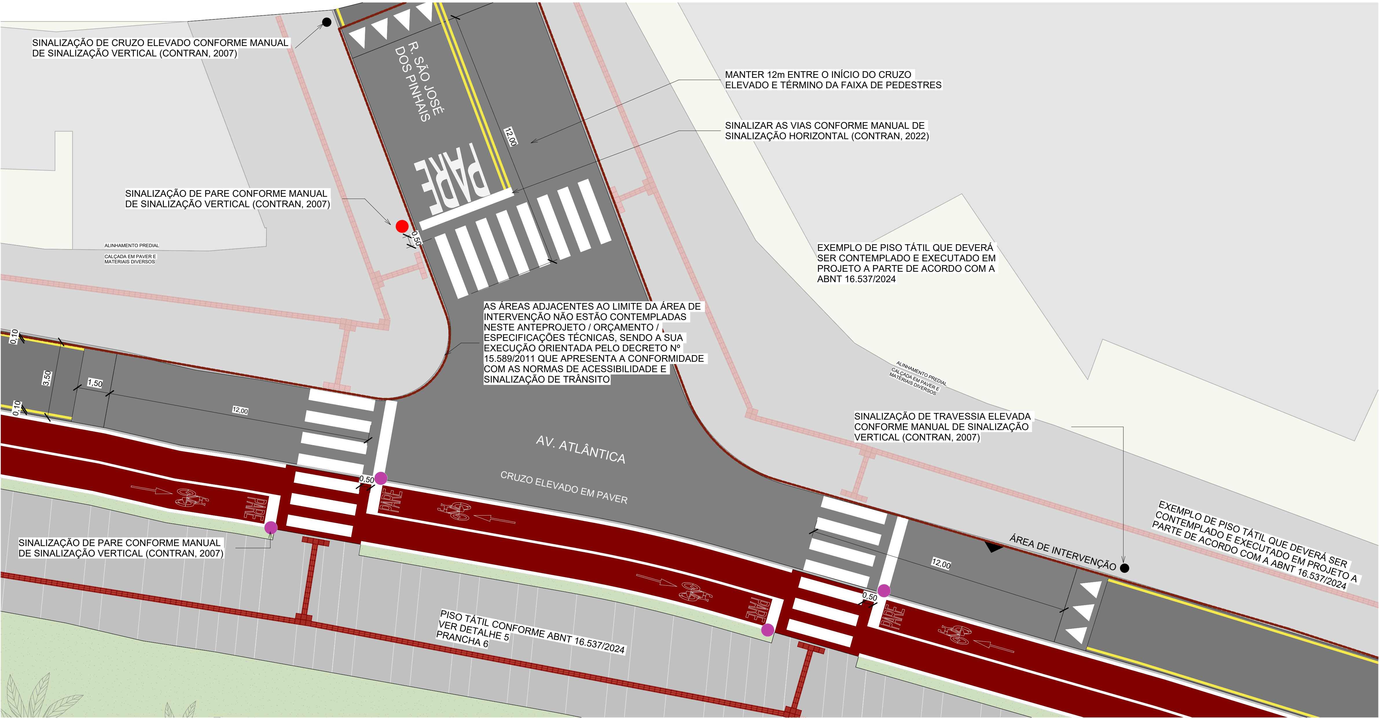
2 ENCONTRO VIÁRIO 2 1 : 100
