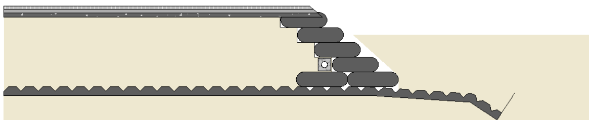
FIGURA 9 – CONTENÇÃO EM GEOTEXTIL
